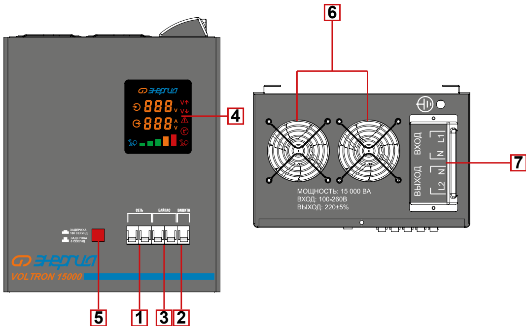
Верхняя панель
